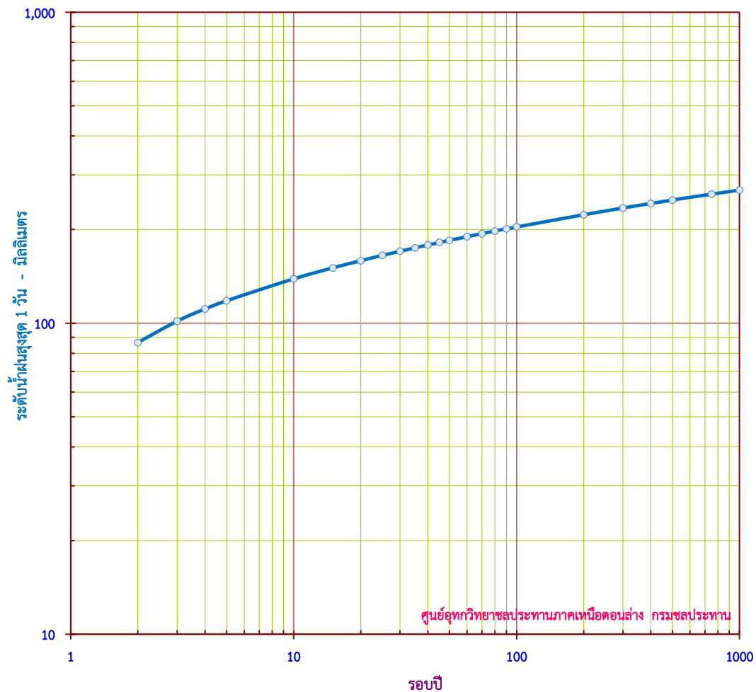
กราฟแสดง ปริมาณน้ำฝนสูงสุด1วัน ขนาดรอบปีต่างๆ สถานี 700151 อ.ท่าปลา จ.อุตรดิตถ์
